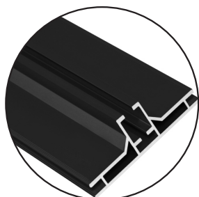
Frame Profiles SKU: VAIL-120DB
